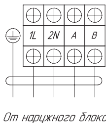
Клеммный терминал внутреннего блока
